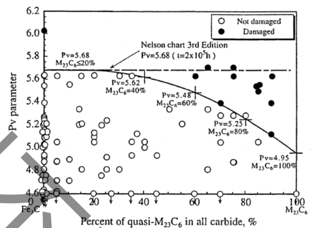
図 4.3 全炭化物中の M_{23}C_6 の割合と P_V 値の関係 [1] （実線は P_V^{cr} を示す。）
