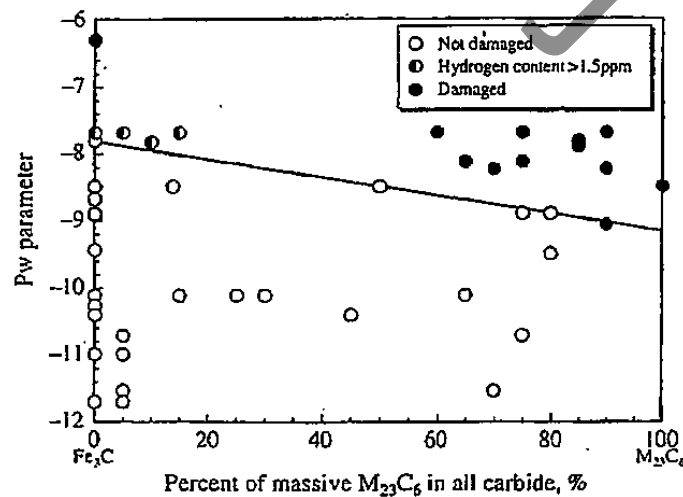
図 4.4 全炭化物中の M_{23}C_6 の割合と P_W 値の関係 [2] （実線は P_W^{cr} を示す。）
