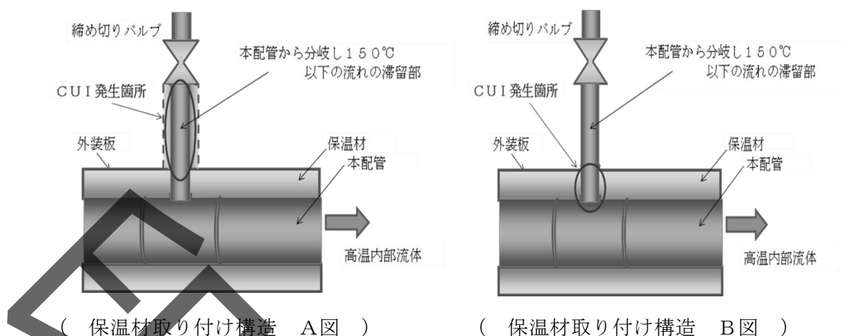
図-13 デッド部（使用停止）配管&温度降下のある配管のCUI
