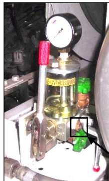
油圧ポンプに取り付けられたヒューズメタル
