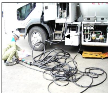
均圧ホース
