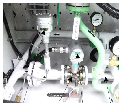
流量計本体 測温抵抗体 整流管 発信装置
