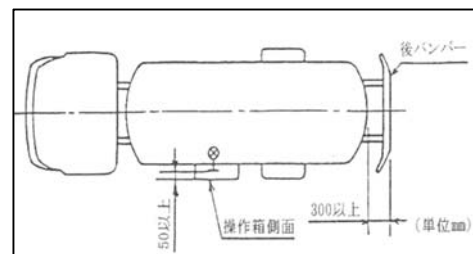
容器と後部バンパとの距離
