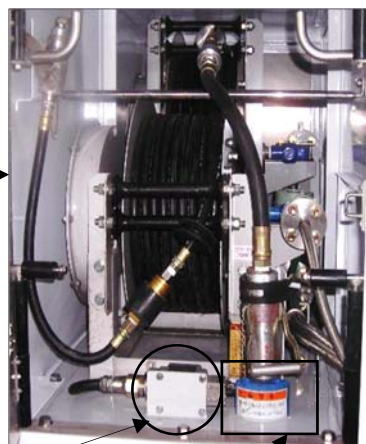
リミットスイッチ セフティカップリング及び受台
