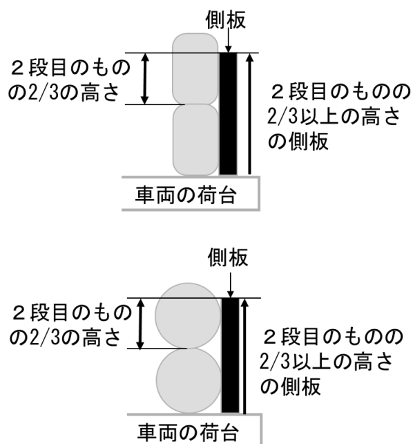
図 充填容器等を２段に積み重ねた場合の側板の高さ（概念図 上：縦積み、下：横積み）
