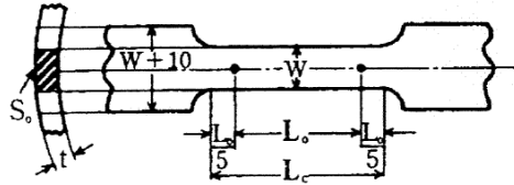
図1 引張試験片の形状
