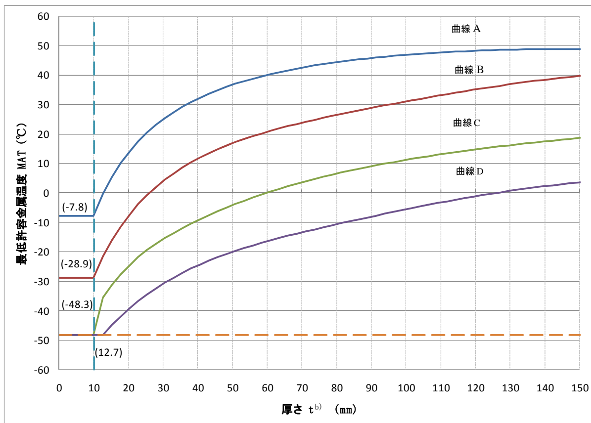
附属書 11 図 1 衝撃試験免除曲線 [1]
