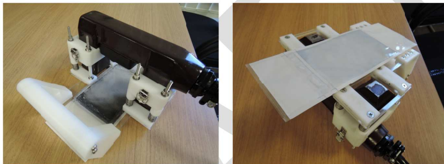
図 B.3－組立後の密閉型磁粉探傷装置（製品例）
