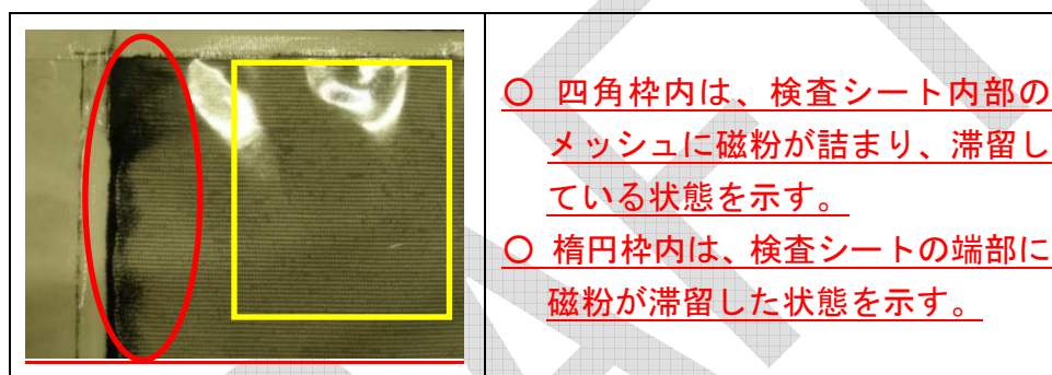
図 B.9—検査シート内に磁粉が滞留している状態（例）
