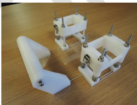
図 B.4ー検査ジグ（構造例） 図 B.5ー検査シート押さえ（製品例）
