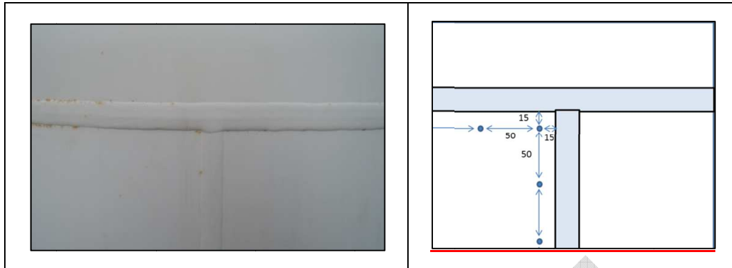
図 B.1ー再塗装を行った履歴がない場合膜厚測定点の例
