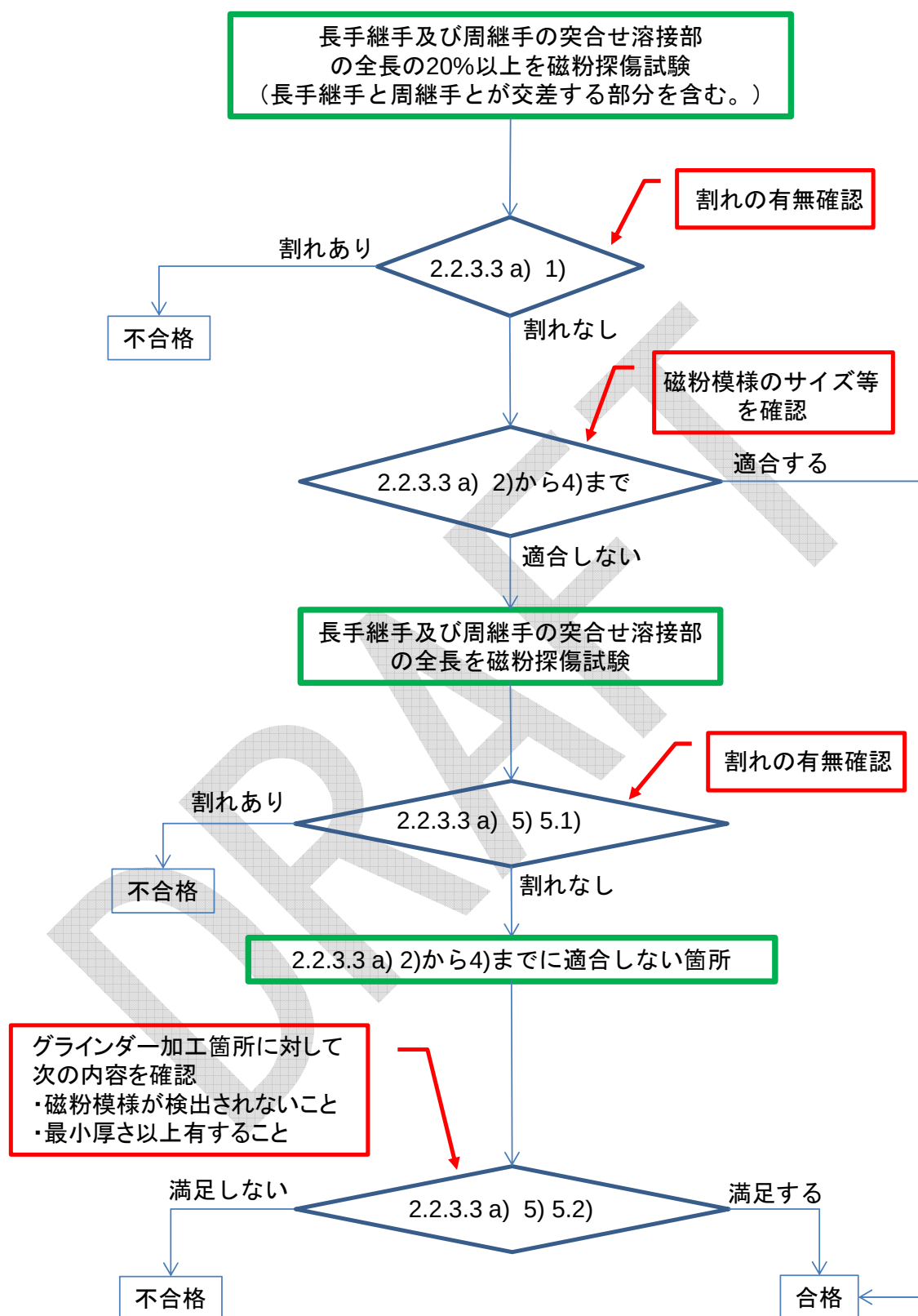
図 3ーバルク貯槽の外面の非破壊検査に係る検査フロー図
